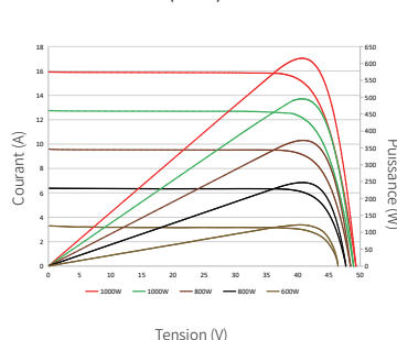
Courbes courant-tension et puissance-tension (615W)
